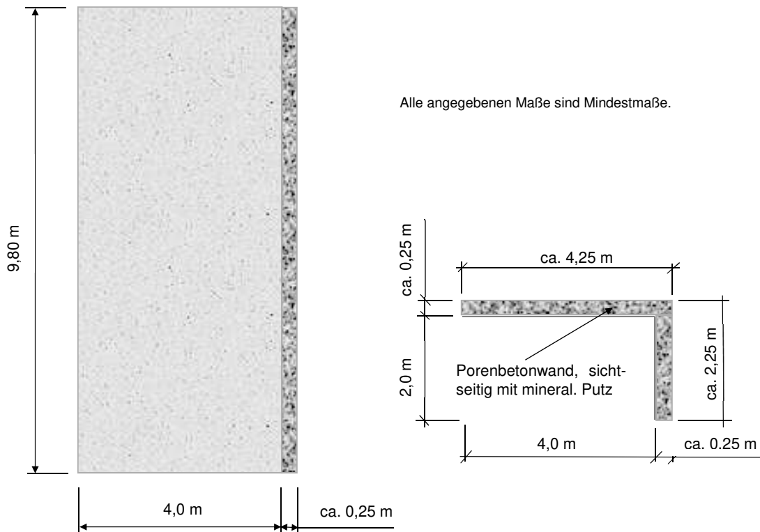
Ansicht des Prüfstandes, Blick auf die Rückwand
