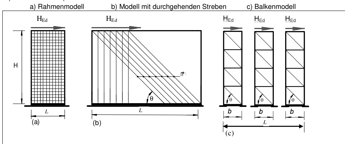
Abb. 1: Statische Modelle für horizontale Scherkräfte H_{Ed}
