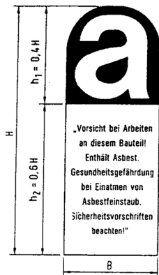
H \cong 50 \text{ mm} B \cong 25 \text{ mm} Bild 1. Kennzeichnung
