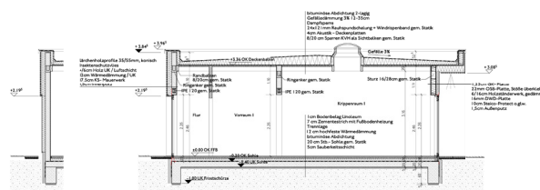
Schnitt B-B
