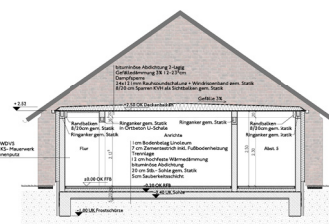
Schnitt A-A
