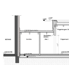
Schnitt C-C
